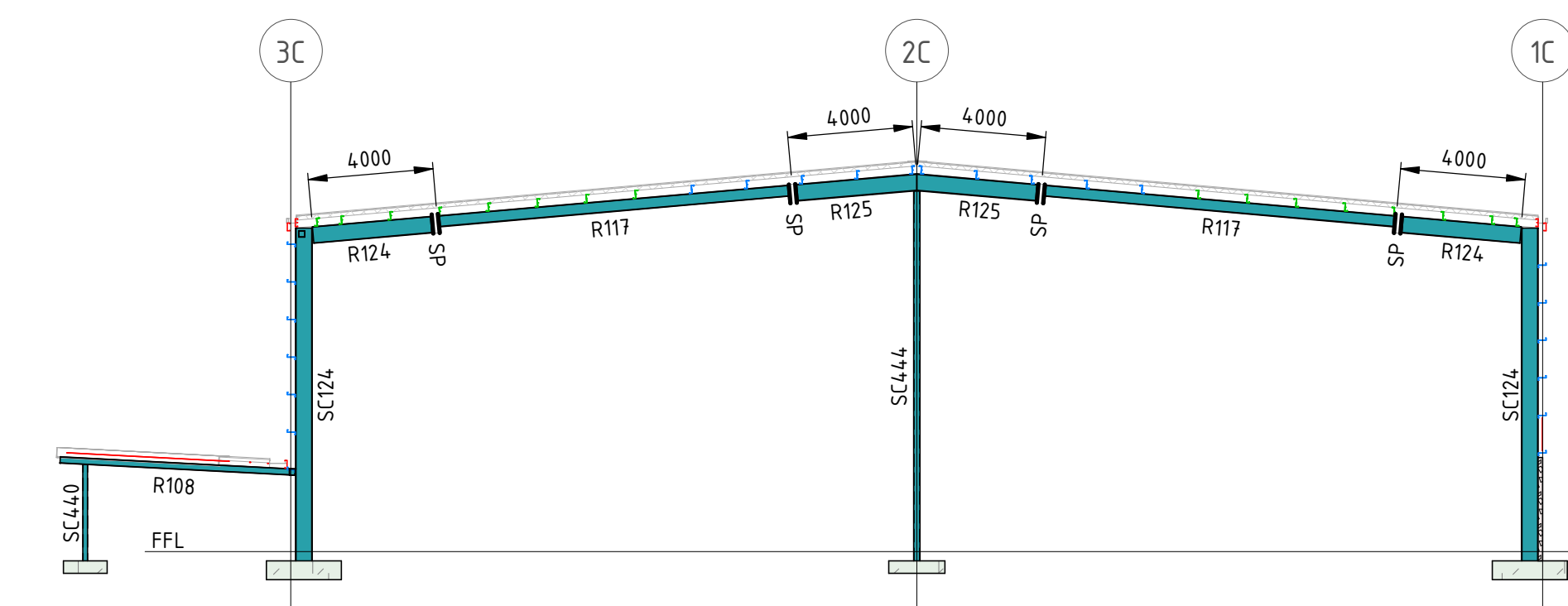
SECTION C6 SCALE 1 : 200 001003
