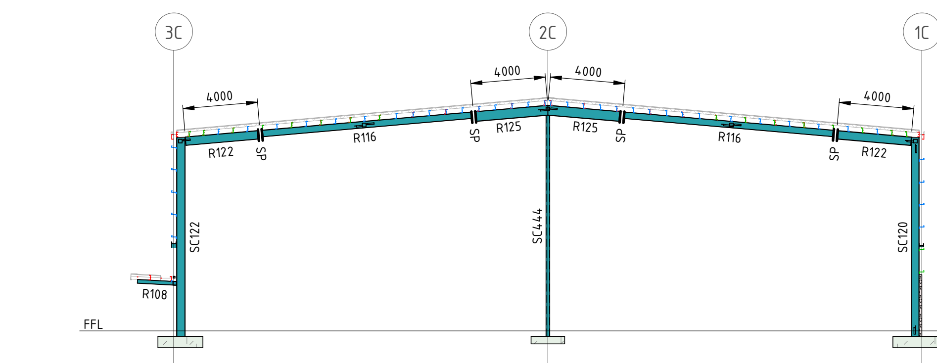
SECTION C8 SCALE 1 : 200 006502
