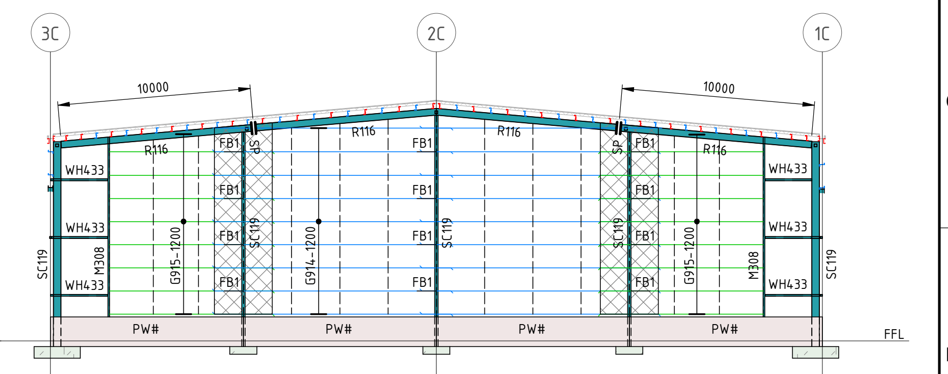
SECTION C10 SCALE 1 : 200 006502
